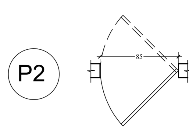
PLANTA ESC. 1:25
