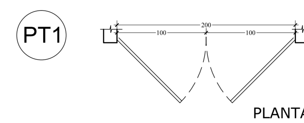
PLANTA ESC. 1:25
